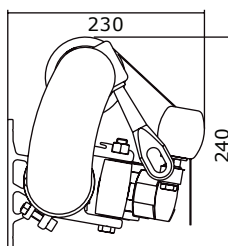
Homlokzati rögzítés
