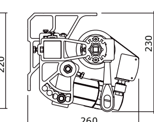
Mennyezeti rögzítés
