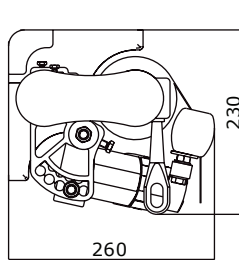
Mennyezeti rögzítés
