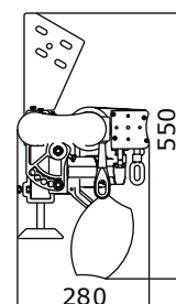
Szarufa rögzítés
