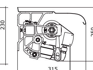
Homlokzati rögzítés védőtetővel
