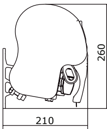
Homlokzati rögzítés
