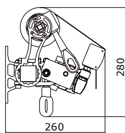
Homlokzati rögzítés
