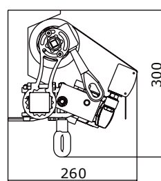
Mennyezeti rögzítés
