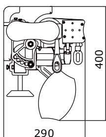
Mennyezeti rögzítés
