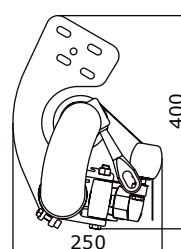
Szarufa rögzítés
