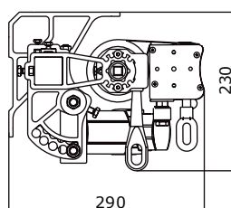
Mennyezeti rögzítés
