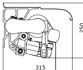
Homlokzati rögzítés védőtetővel
