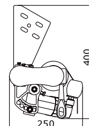
Szarufa rögzítés
