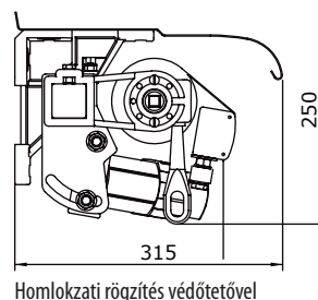
Homlokzati rögzítés védőtetővel
