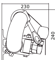
Homlokzati rögzítés
