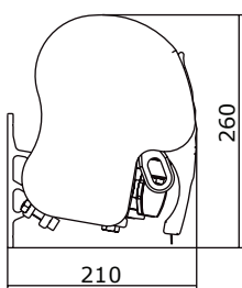
Homlokzati rögzítés
