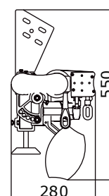
Szarufa rögzítés
