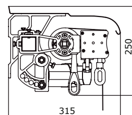
Homlokzati rögzítés védőtetővel
