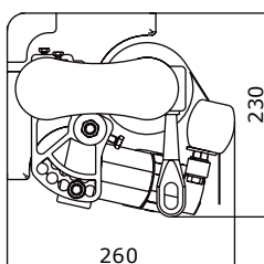
Mennyezeti rögzítés
