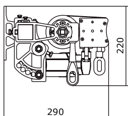
Homlokzati rögzítés
