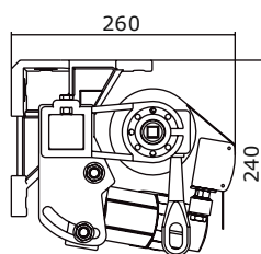
Mennyezeti rögzítés
